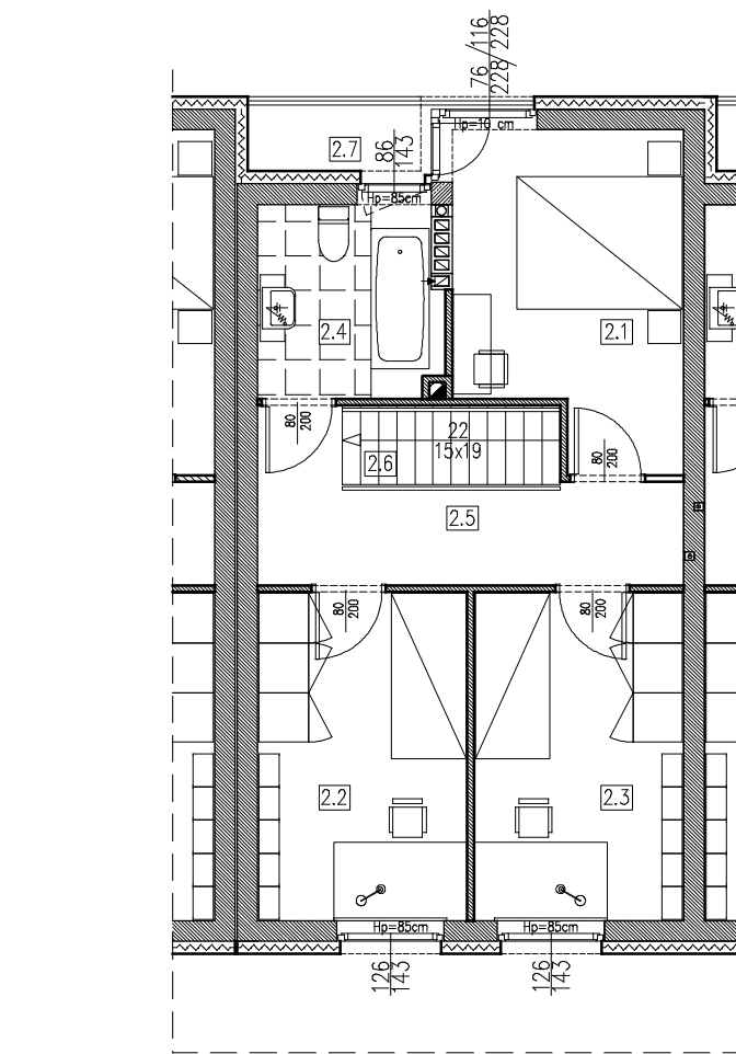
KONDYGNACJA +2
