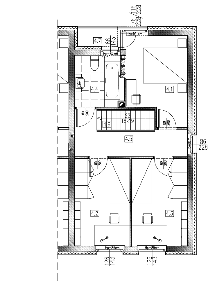
KONDYGNACJA +2
