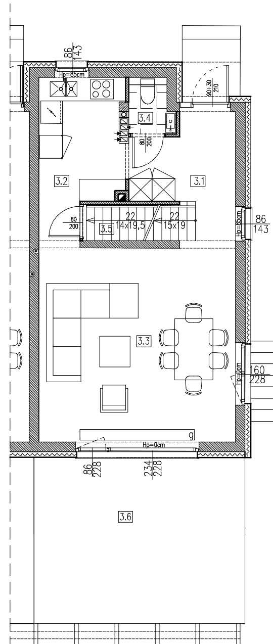
KONDYGNACJA +1
